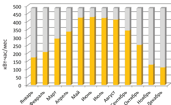
Количество тепла, которое выработает система в Южных регионах Украины (годовая выработка системы составляет 3 947кВт-час)
