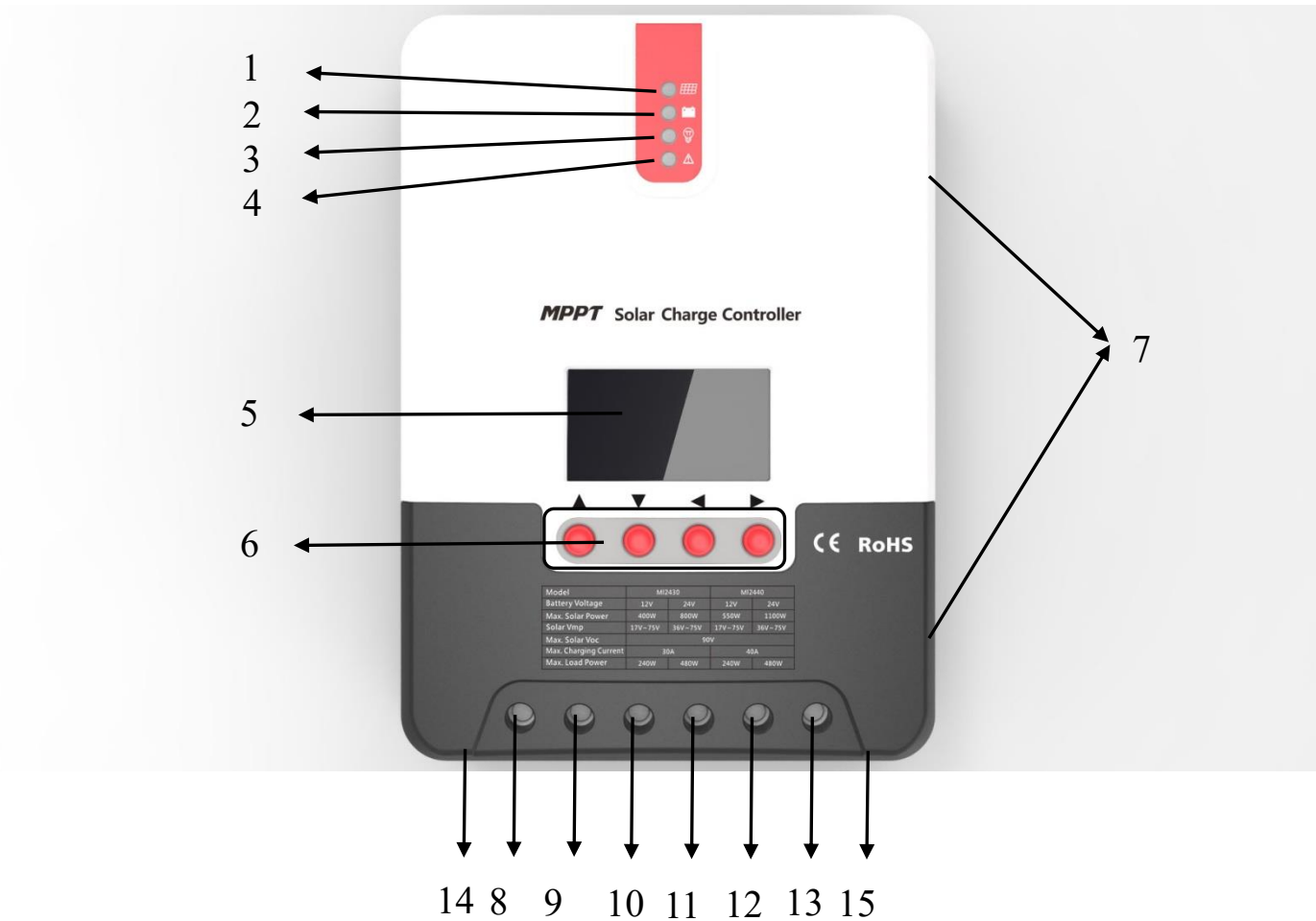
Рис. 1.1 – Елементи контролеру
