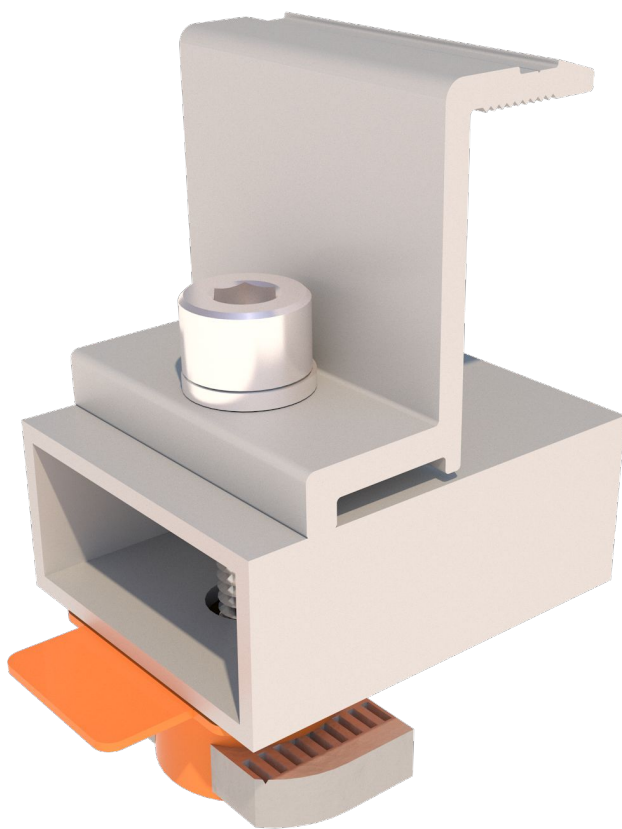
Z-подібний прижим Bifacial
